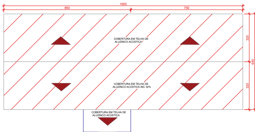
PLANTA DE COBERTURA
